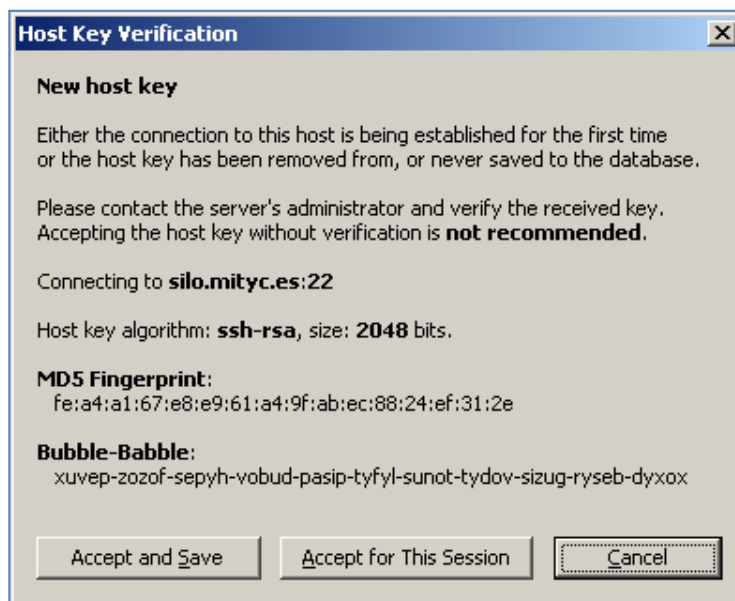
Figura 12 - Tunnelier: Aceptar certificado de silo.mityc.es
